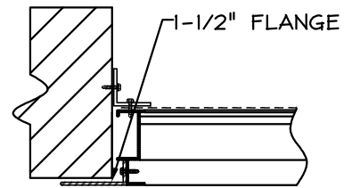
(EXTERIOR) FLANGE FRAME
